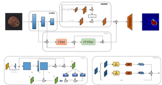
图 1 多层次特征融合网络图
