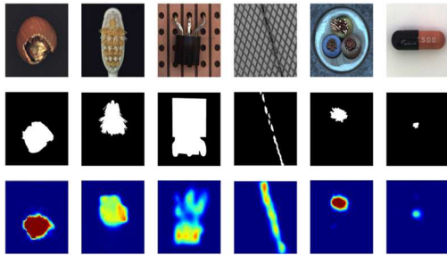
图 5 异常检测可视化图
