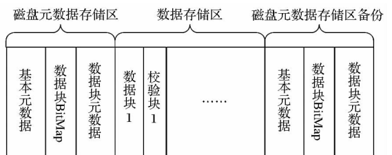
图 3 FlatLFS 中的磁盘数据组织框架
