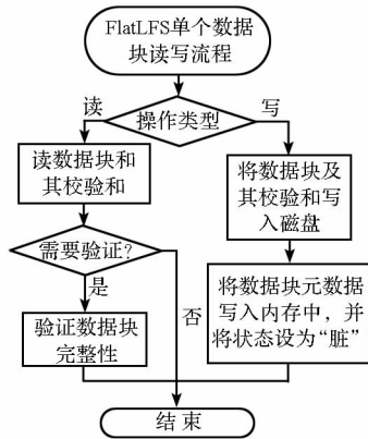
(c) FlatLFS 单个数据块读写流程
