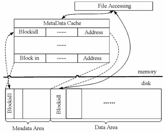
图 2 FlatLFS 数据块定位
