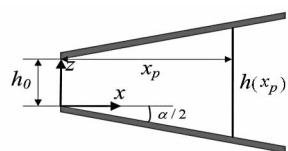
图 4 极板张角示意图
