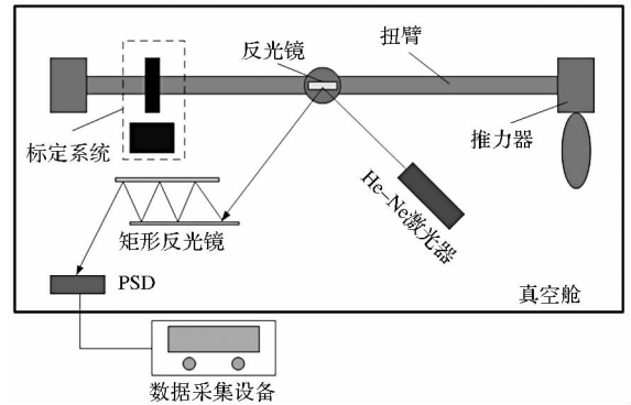
图7 扭摆工作原理图
