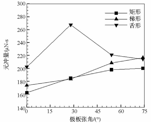
图 10 元冲量随极板张角的变化 Fig. 10 Impulse bit over flare angle
