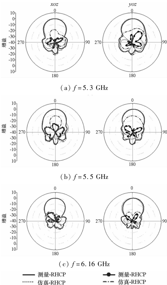
图 7 微带贴片阵列不同频率点上 xoz 和 yoZ 面上的仿真及测量方向图
