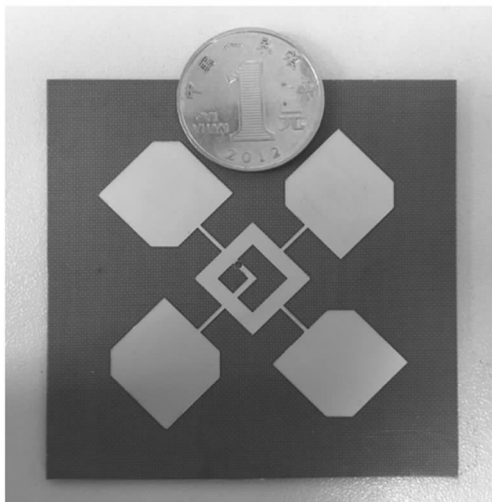
图 2 贴片阵列加工的实物照片
