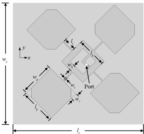
图 1 阵列天线结构及尺寸示意图
