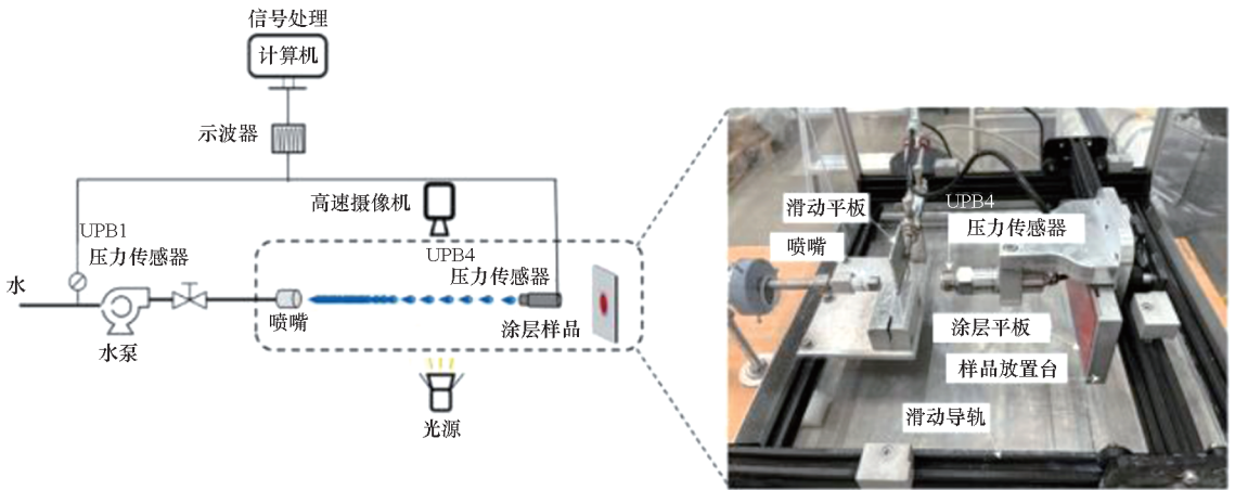
图 29 脉动水射流试验机的示意图和实际视图 [94]
