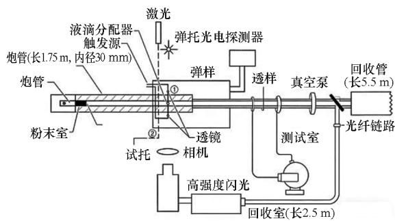
图 19 GRCI 水凝物撞击装置 [28]
