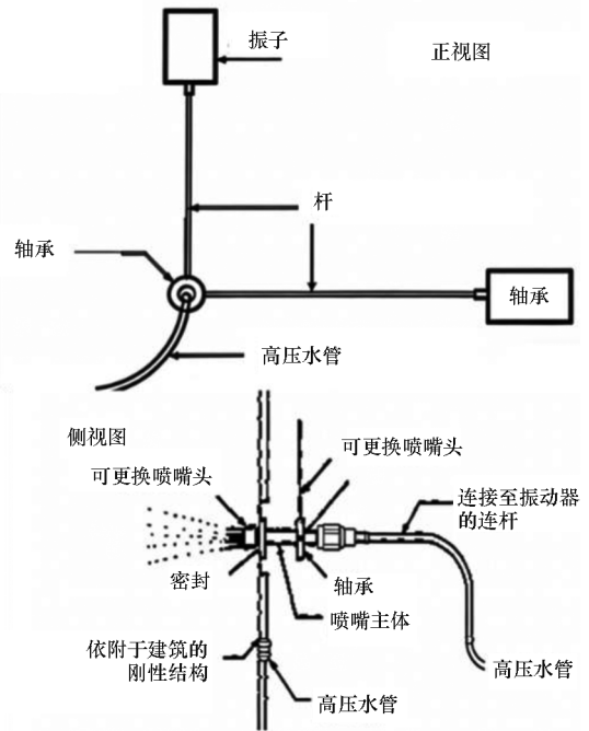
(b) 振动喷嘴连接示意图
