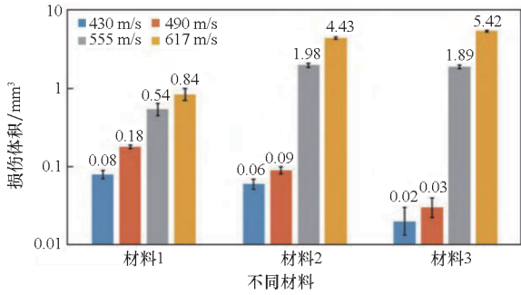
图 5 损伤体积随冲击速度的变化 [20]
