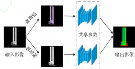
图 3 一致性正则化的原理
