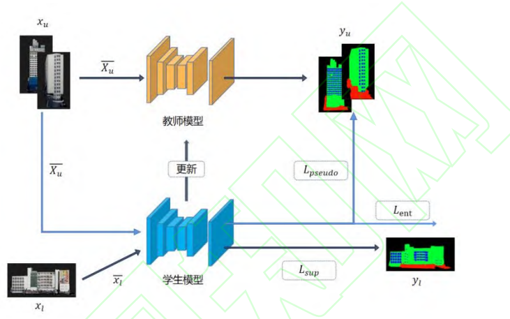
图 1 SS_CC 模型框架图
