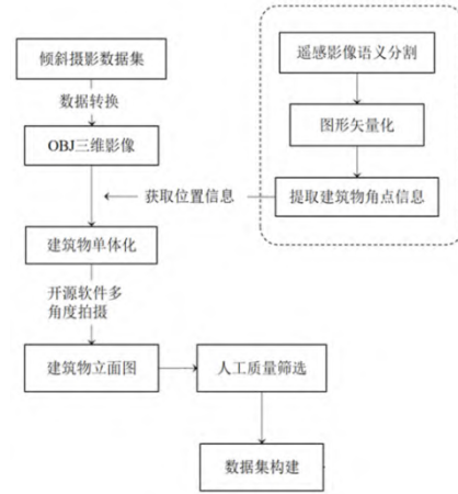
图 4 建筑物立面提取方法
