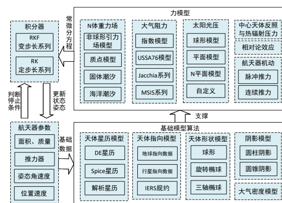
图 6 ATK 高精度轨道预报模型组建设计
