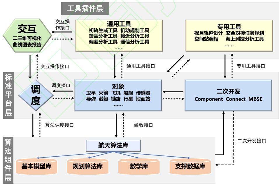
图 4 ATK 分层组件式架构组成
