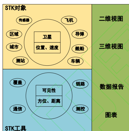
图 5 基于本体论的 STK 功能框架描述
