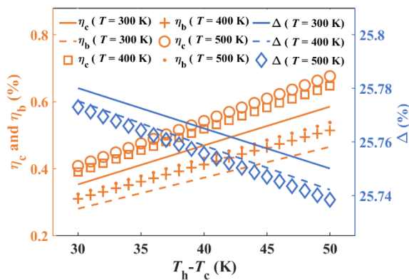
图 11 扩展平面热聚集器对于热点转换效率提升的理论结果 [18]
