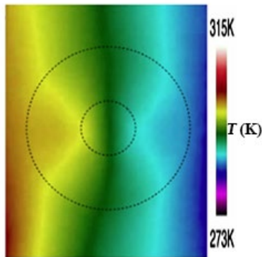
图3 热聚集器的实验结果 [10]
