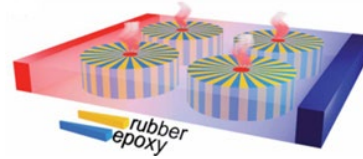
图8 基于热聚集器实现热电转换效率提升 [16]
