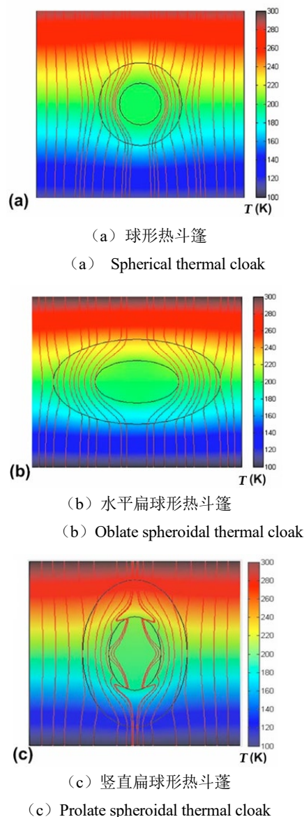
图1 不同几何构型下的热斗篷 [1]
