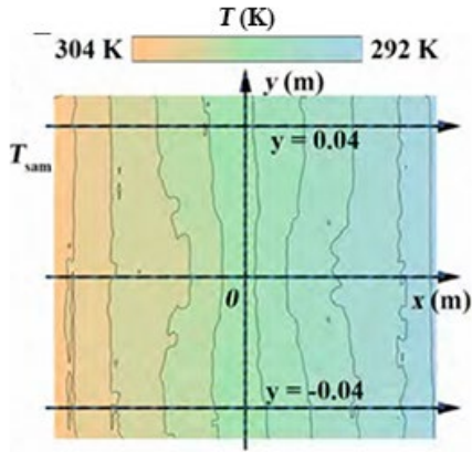
图 10 扩展平面热聚集器的实验结果 [18]
