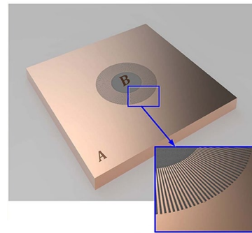
图9 基于热聚集器实现局部加热 [17]
