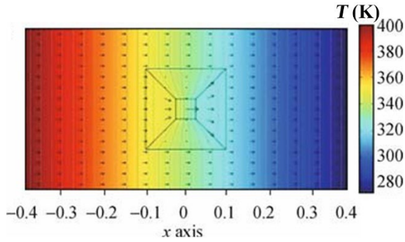
图2 热聚集器的提出及模拟结果 [9]
