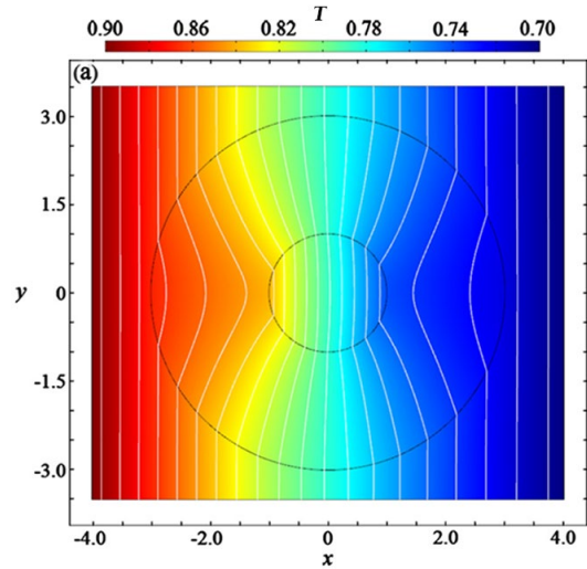
(a) 可切换聚集器的有限元模拟结果(聚集器状态)
