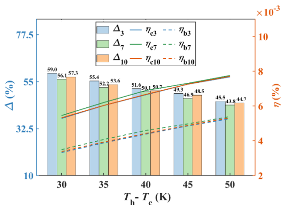
图 12 扩展平面热聚集器对于热点转换效率提升的实验结果 [18]
