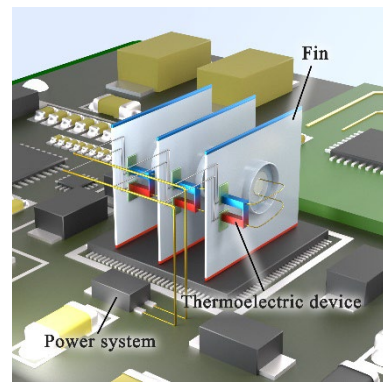
图 13 基于热聚集器实现芯片散热 [18]
