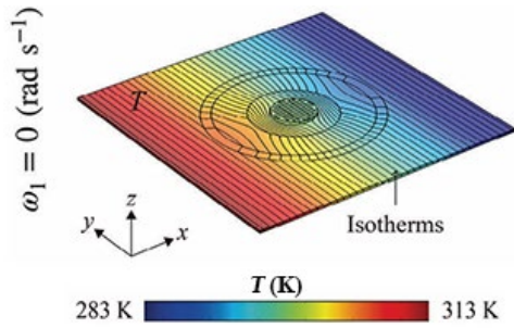
图7 基于深度学习热聚集器的模拟结果 [15]
