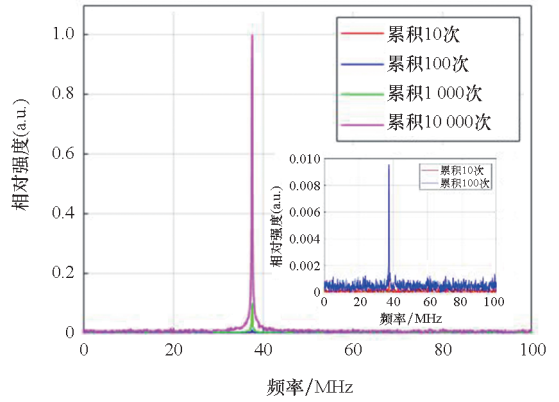
图 8 11 μs 脉冲累积 10 次、100 次、1 000 次和 10 000 次后的频域信号
