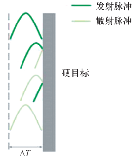
图 1 激光脉冲被硬目标散射的过程示意图
