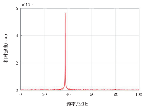
图 9 硬目标前一个大气距离门内的频谱信息
