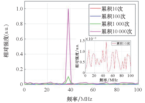
图 6 400 ns 脉冲累积 10 次、100 次、1 000 次和 10 000 次后的频域信号
