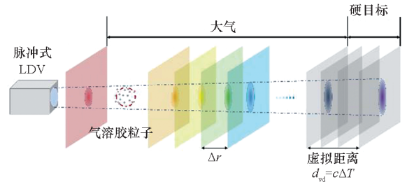
图 2 脉冲式 LDV 时域回波信号模型示意图
