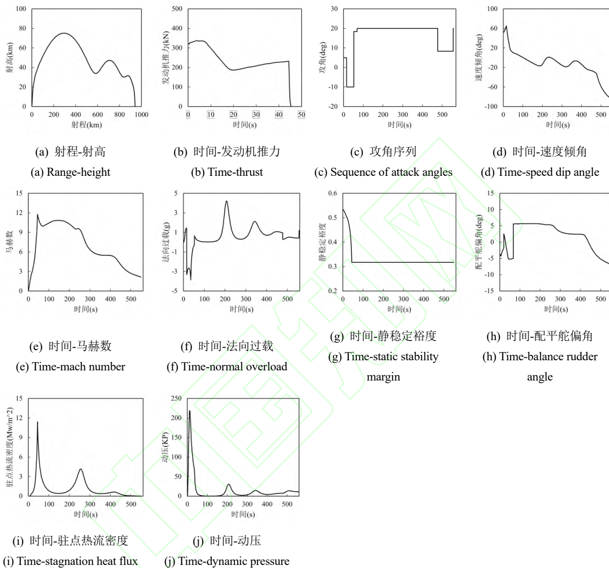
图3 初始方案飞行性能曲线图
