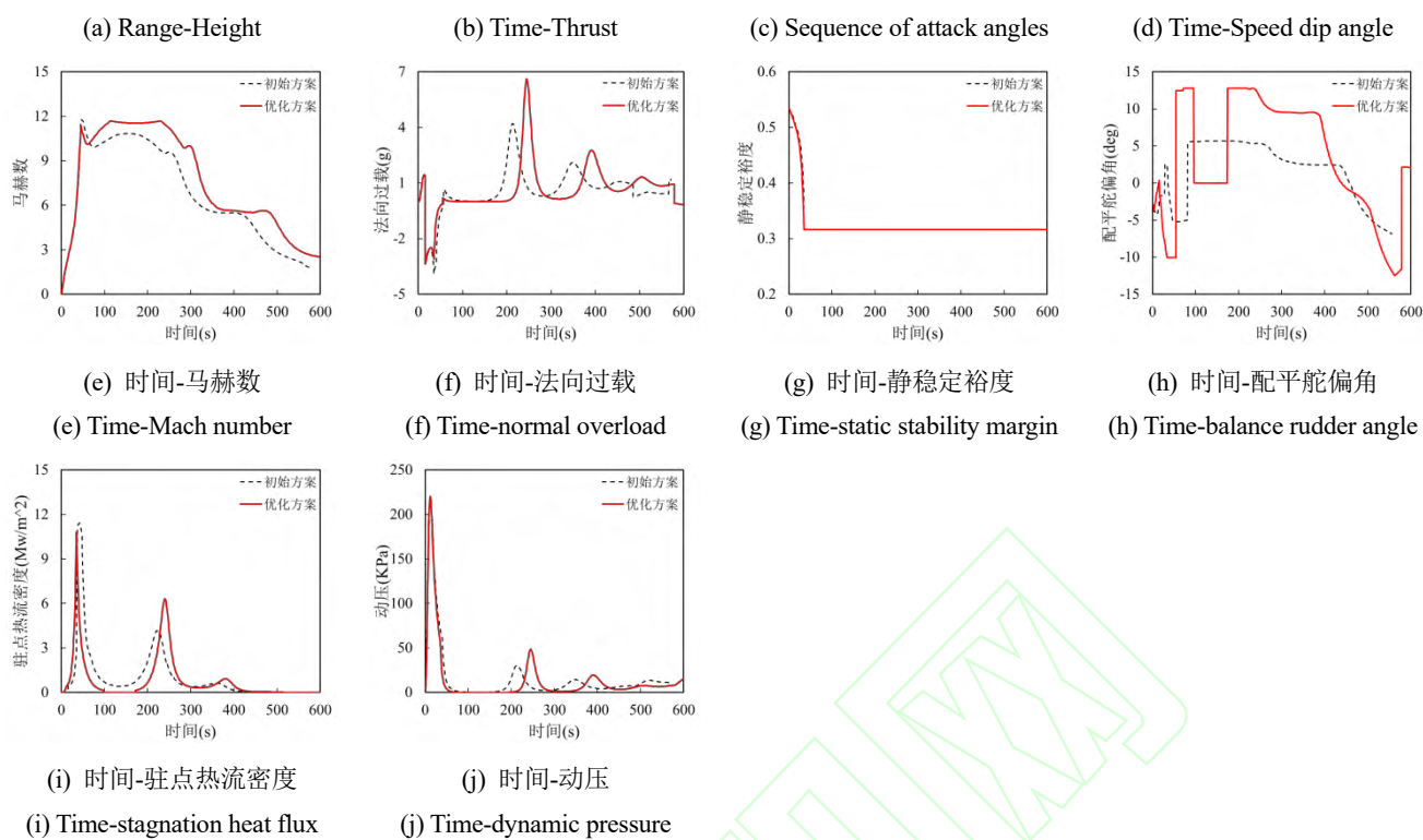
图 7 初始方案与优化方案飞行性能比较
