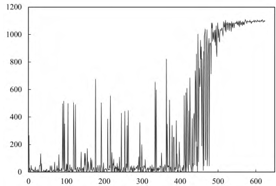
图6 目标函数迭代过程
