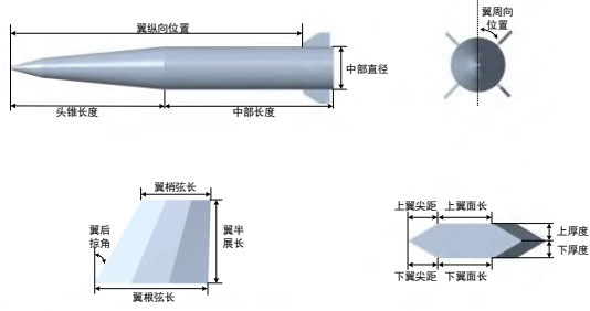
图1 远程制导火箭几何结构示意图
