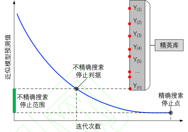
图5 基于不精确搜索的采样过程示意
