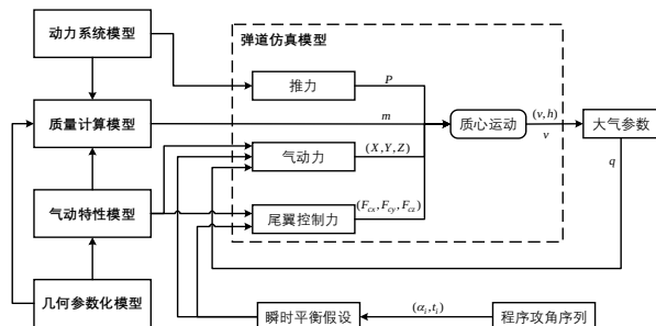
图2 多学科仿真流程示意图
